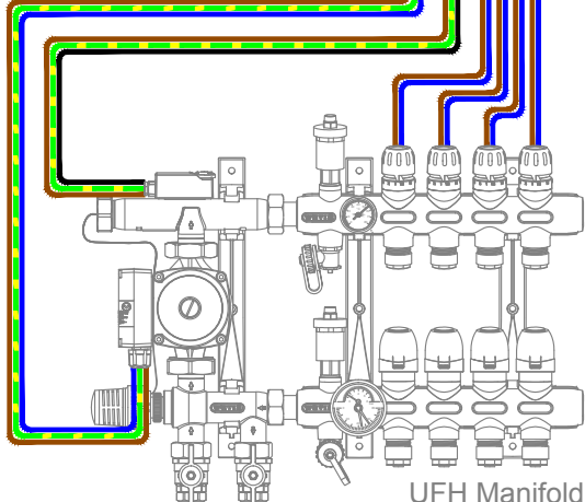
UFH Manifold
