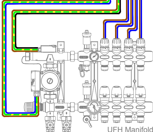
UFH Manifold
